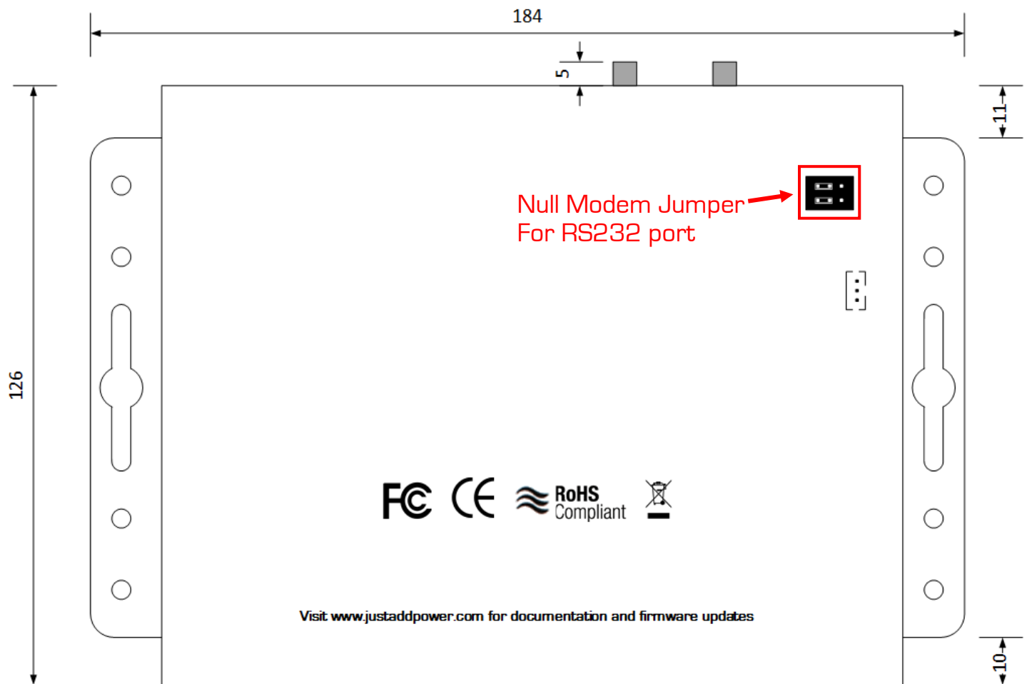
717HIFI Bottom
